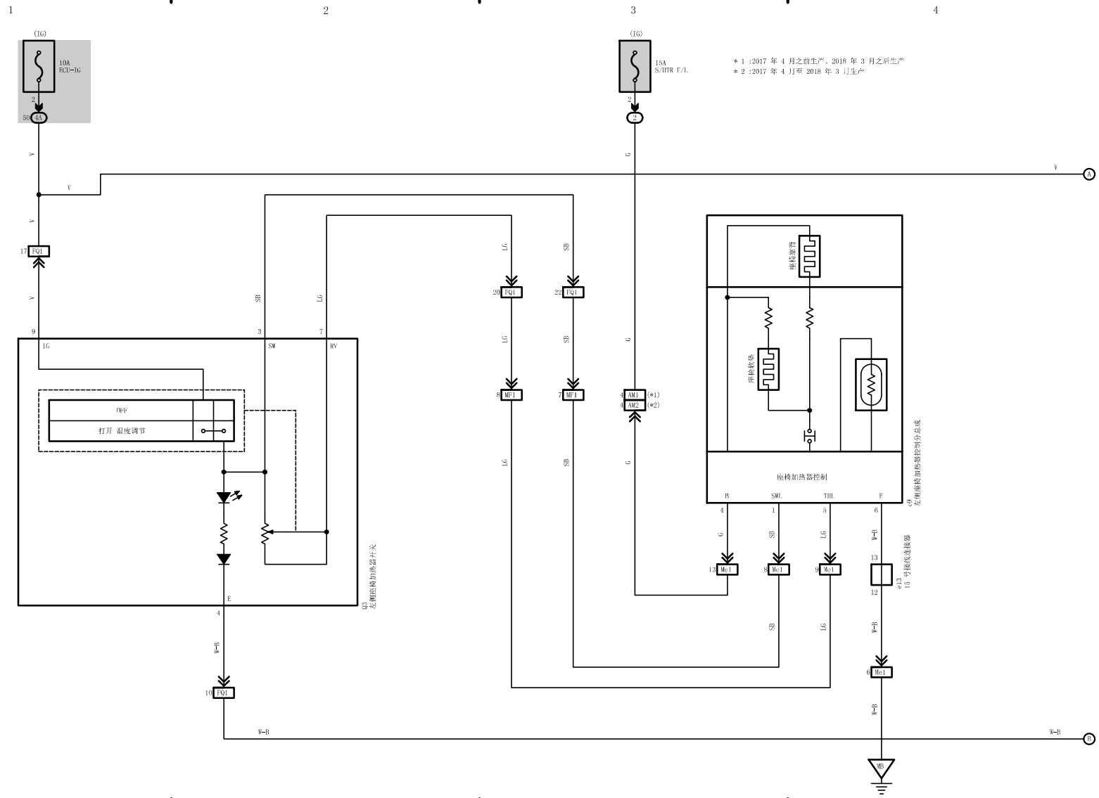
座椅加热器（不带座椅温度控制的前座椅）
